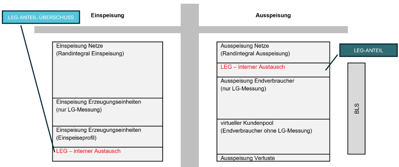
Abbildung 13 Netzbilanzierung mit LEG
